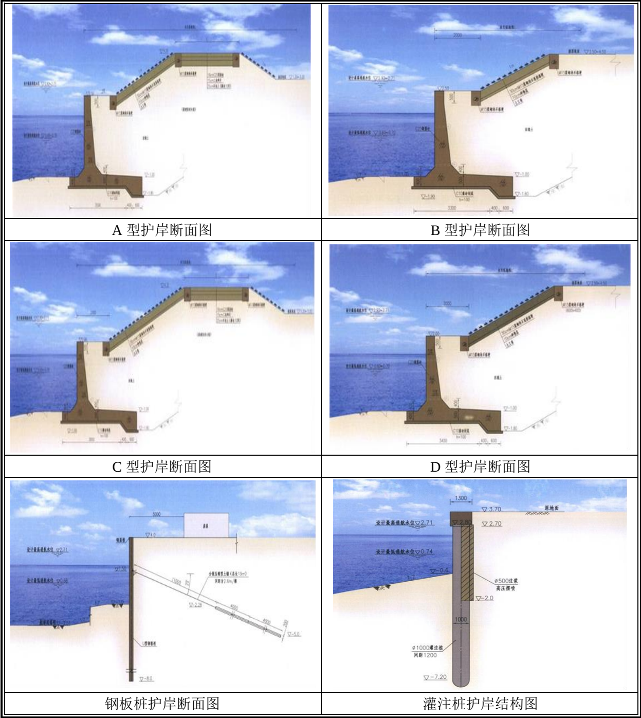
图 2.3-1 典型护岸断面图
